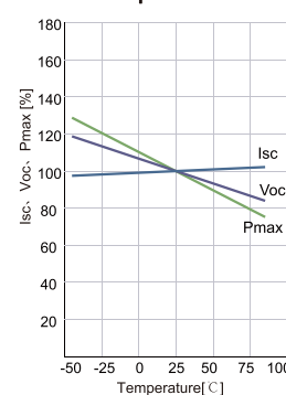
Isc, Voc, Pmax-Temperature Curve
